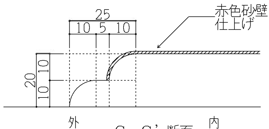
C-C' 断面
