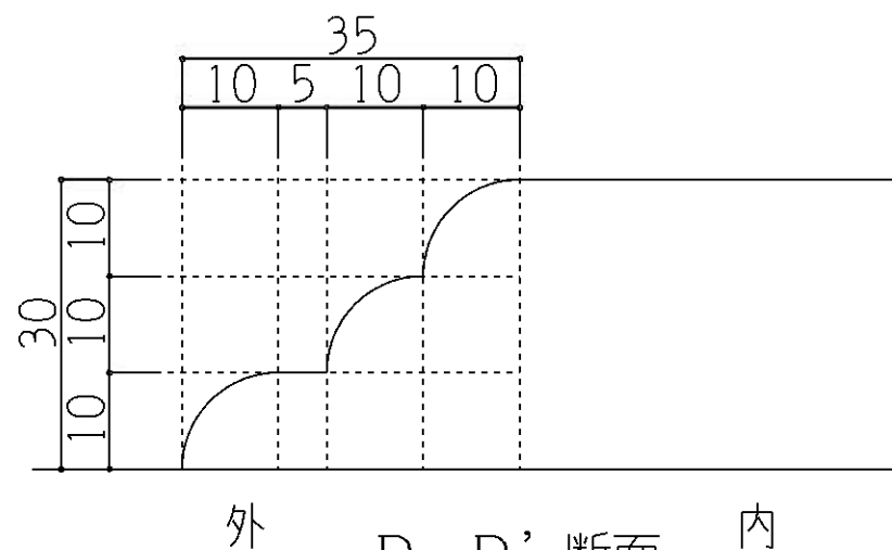
D—D' 断面
