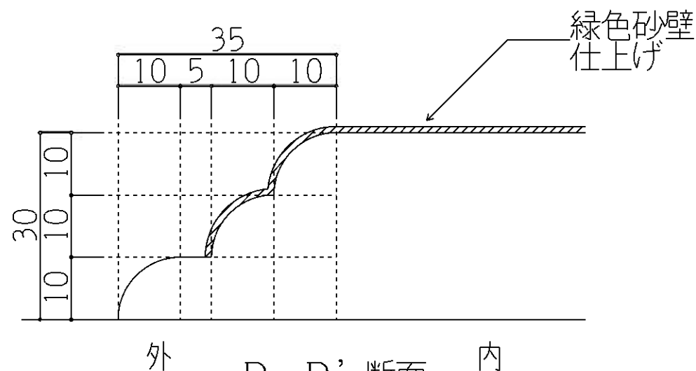
D-D' 断面
