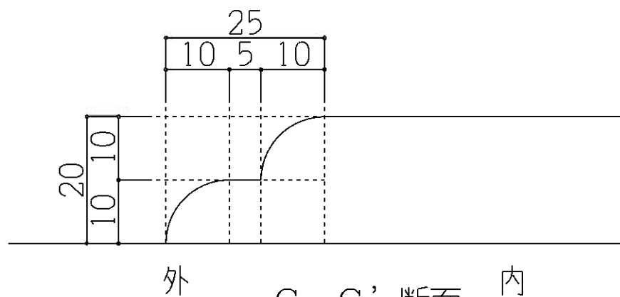
C—C' 断面
