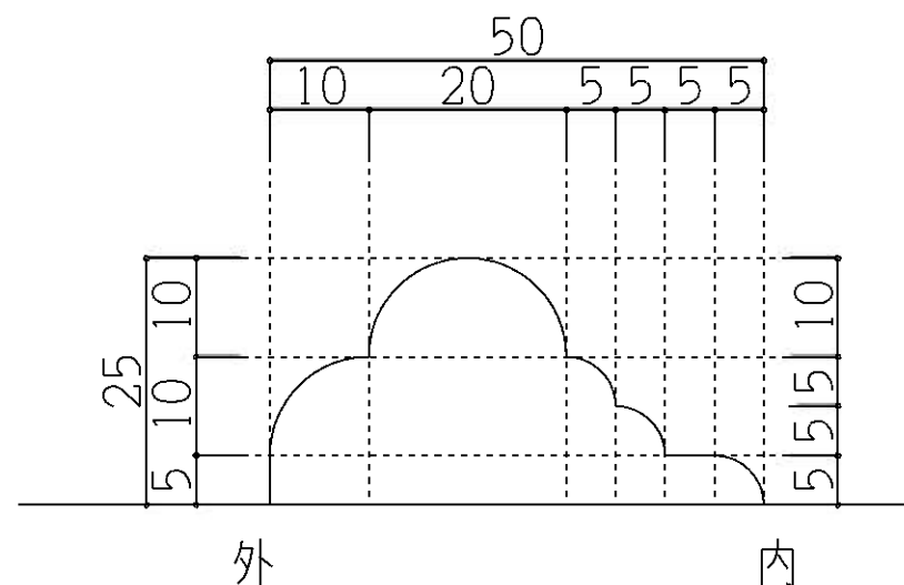
B-B' 断面
