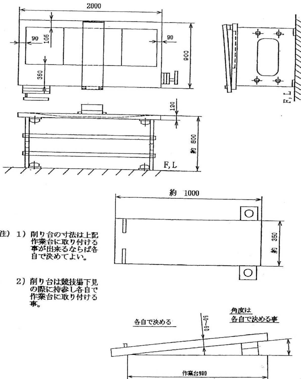
作業台および削り台の図
