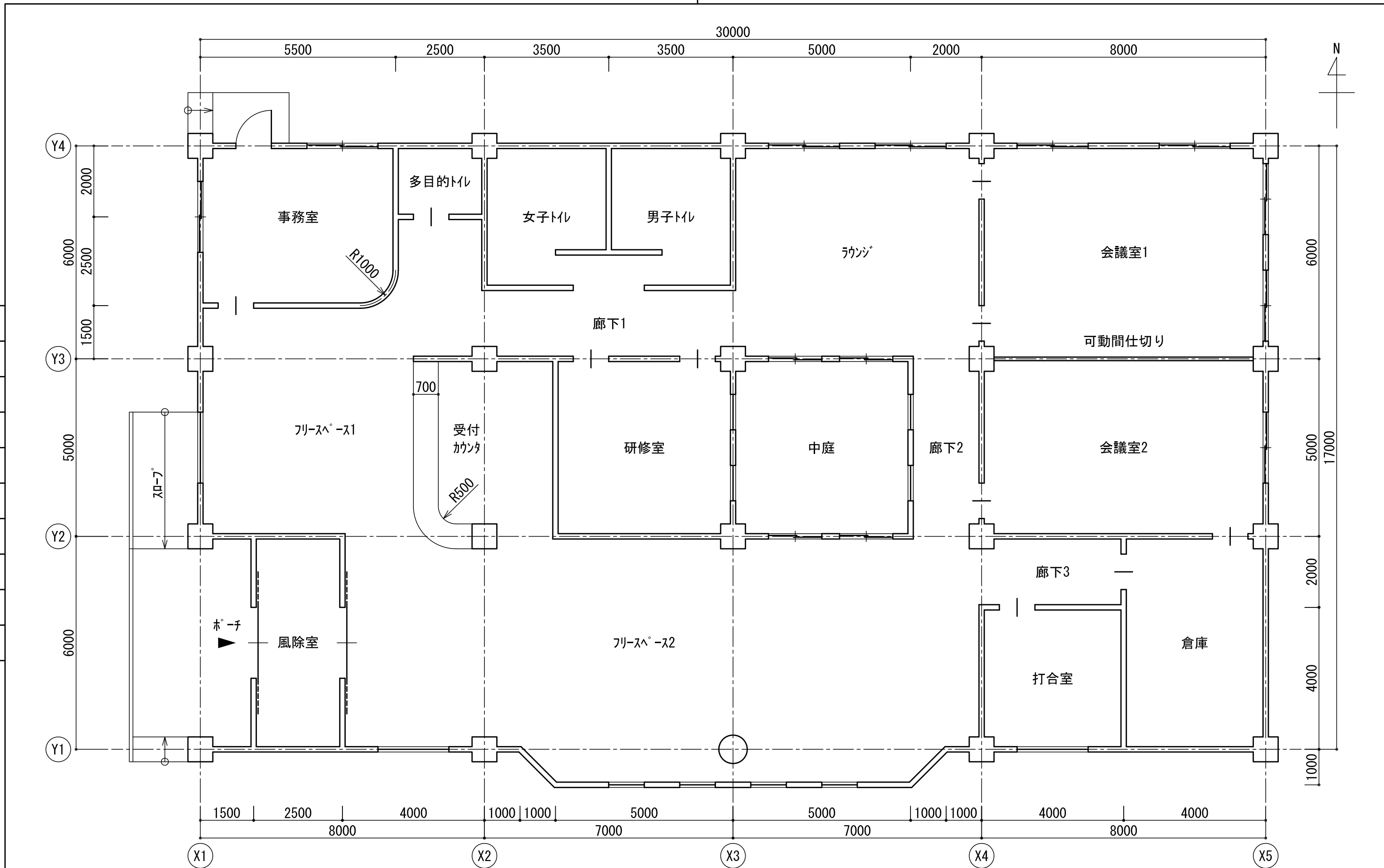
平面図 S=1:100
