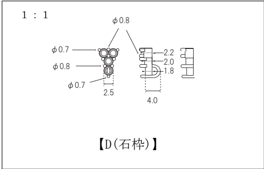
【A/B/C/D/E部接続部裏面拡大】
