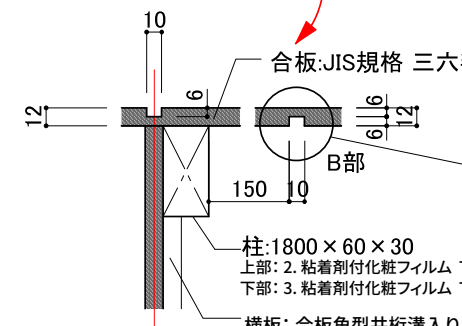
A部詳細図 1/5
