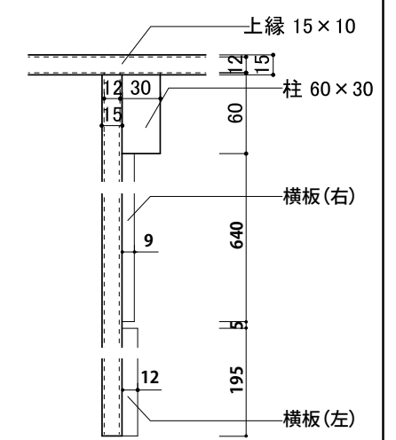
柱取り合い部 伏図 1/5
