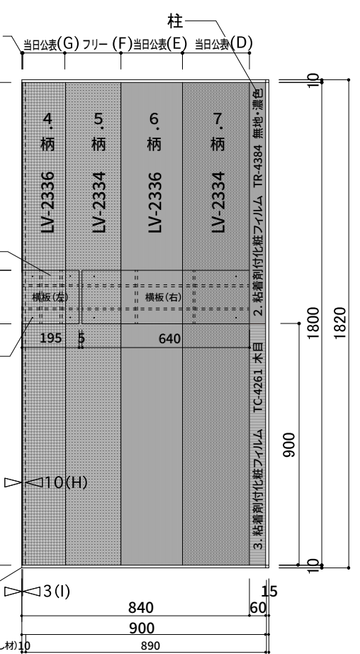
B面 ビニール壁紙 側面図 1/20
