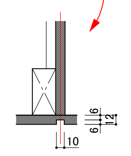
A面 目地部詳細図 1/5
