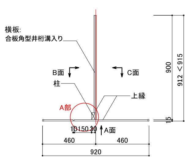
平面図 1/20
