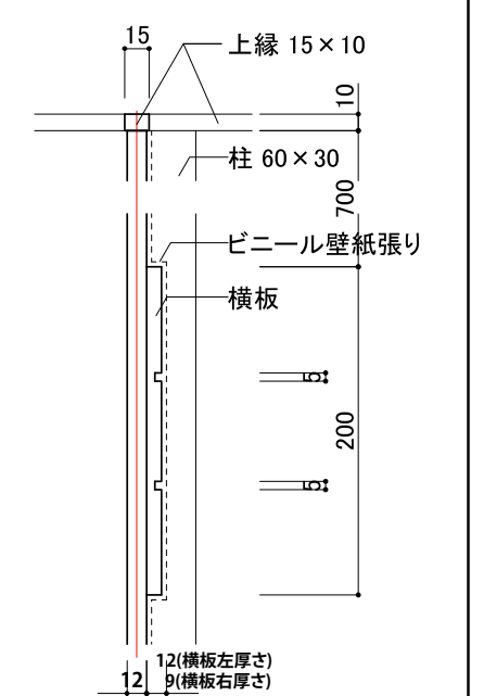
横板部断面図 1/5
