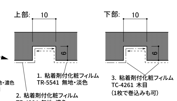
B部詳細図 1/1
