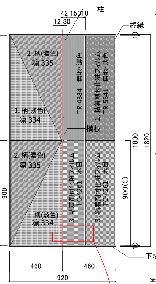
C面 紙壁紙 ⇄ B面 粘着剤付化粧フィルム 背面図 1/20
