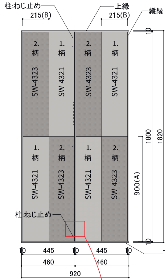
A面 布壁紙 立面図 1/20
