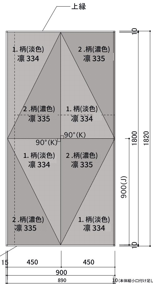
C面 紙壁紙 側面図 1/20
