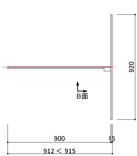
平面図 1/20
