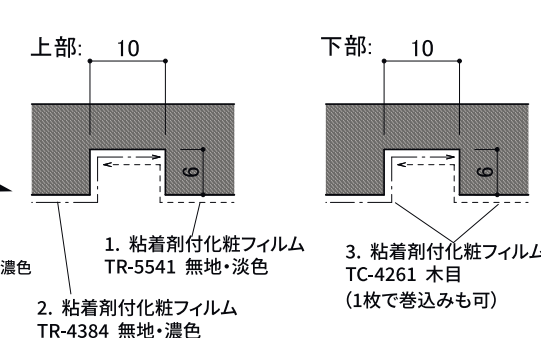
B部詳細図 1/1
