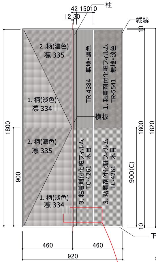
C面 紙壁紙 背面図 1/20 B面 粘着剤付化粧フィルム 背面図 1/20
