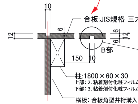
A部詳細図 1/5
