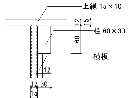
柱取合い部 伏図 1/5
