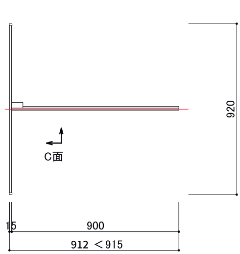
平面図 1/20
