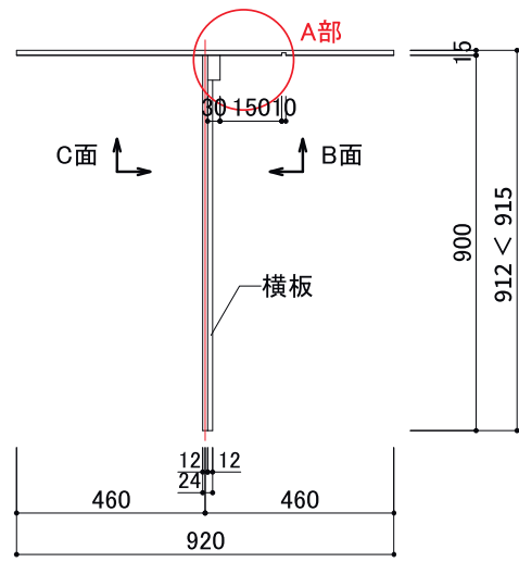
平面図 1/20
