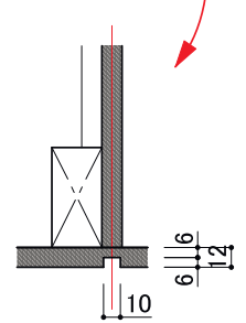
A面 目地部詳細図 1/5
