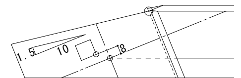
⑫化粧隔木ほぞ詳細図
