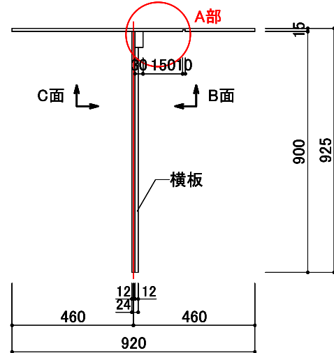
平面図 1/20
