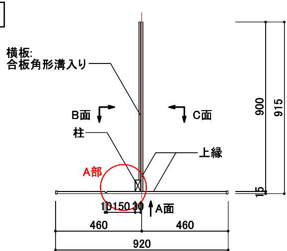
平面図 1/20
