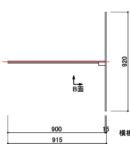
平面図 1/20
