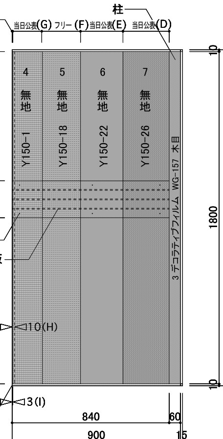
B面 ビニール壁紙 側面図 1/20
