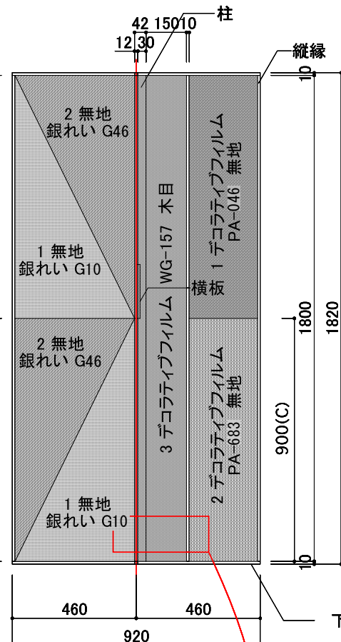
C面 紙壁紙 B面 デコラティブフィルム 背面図 1/20
