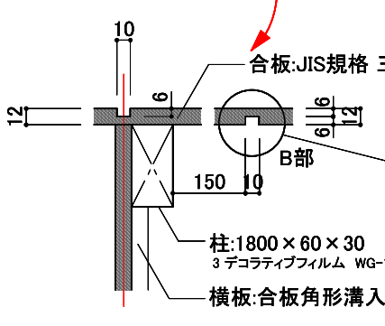
A部詳細図 1/5
