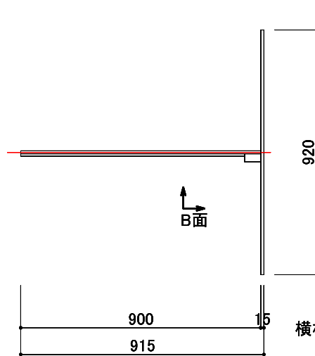
平面図 1/20
