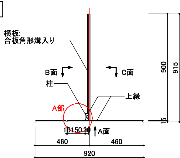
平面図 1/20
