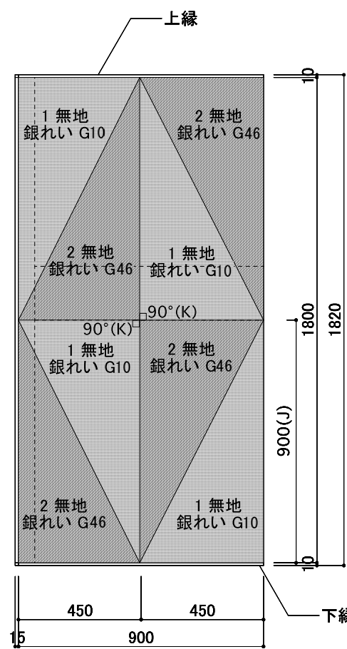
C面 紙壁紙 側面図 1/20
