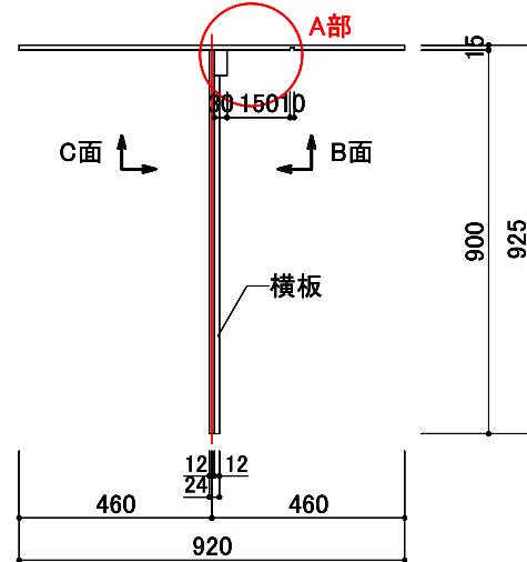
平面図 1/20
