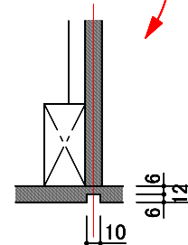
A面 目地部詳細図 1/5
