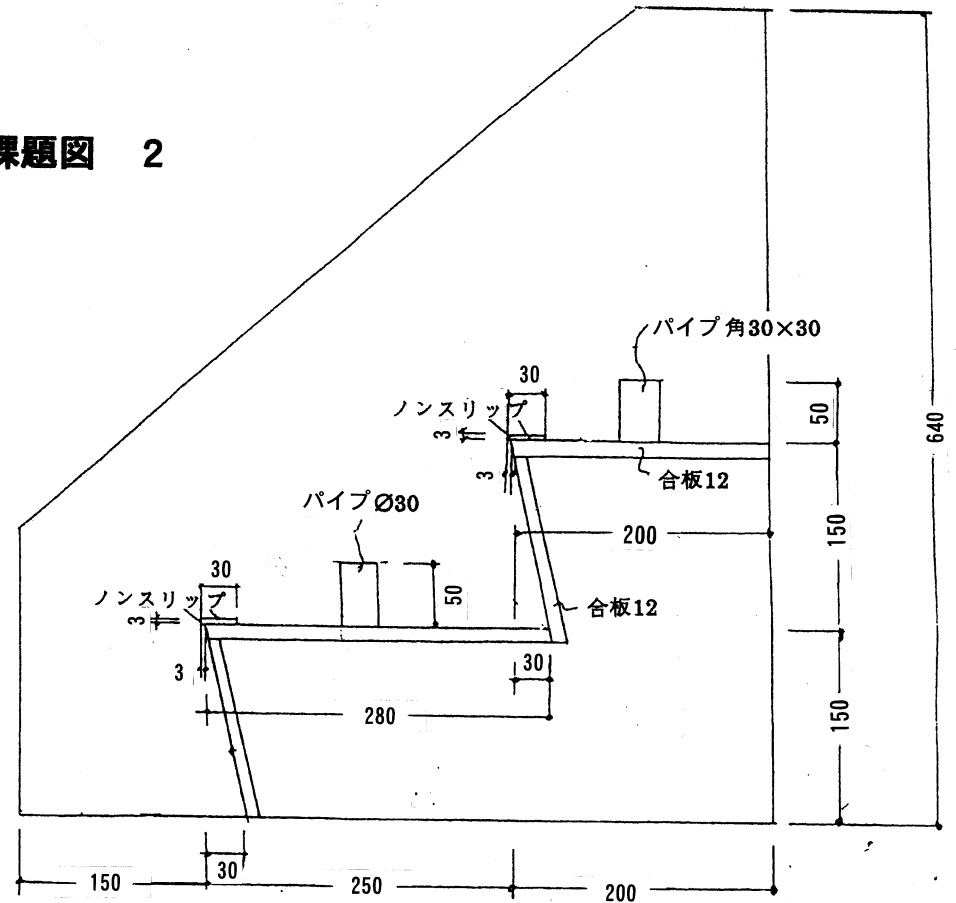
A - A 断面
