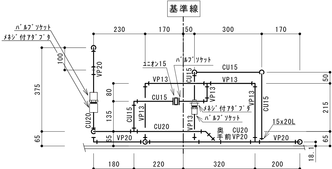
E-E' 立面図 S:1/10
