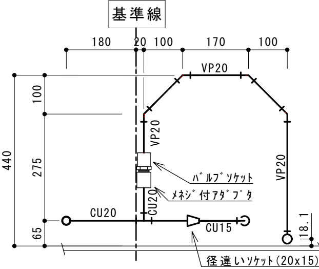
C-C' 断面図 S:1/10
