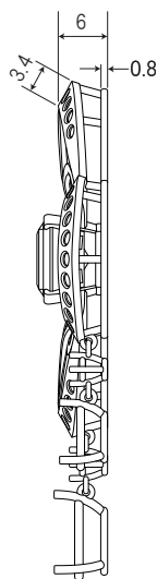
【右側面図】
