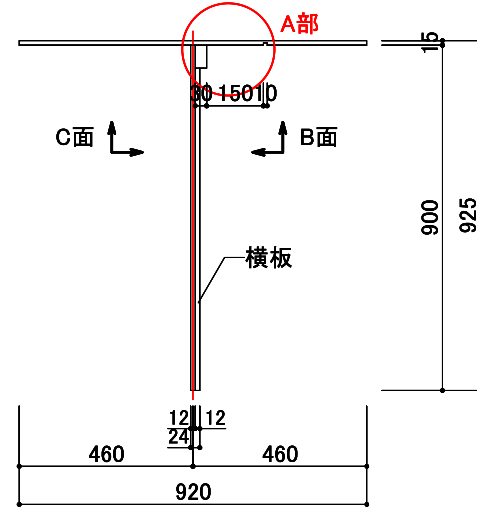
平面図 1/20
