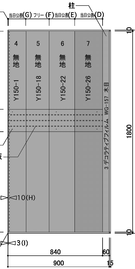
側面図 1/20
