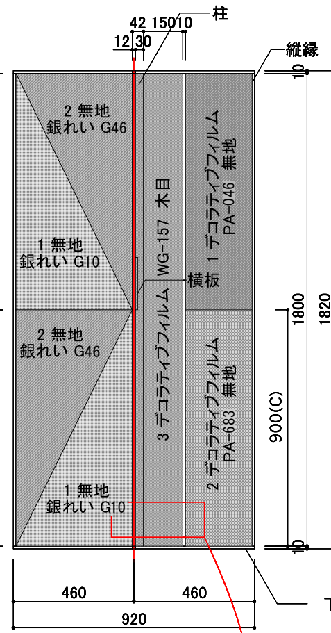
背面図 1/20
