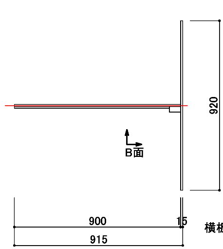
平面図 1/20
