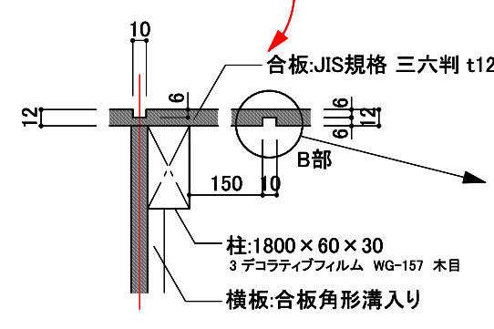
A部詳細図 1/5
