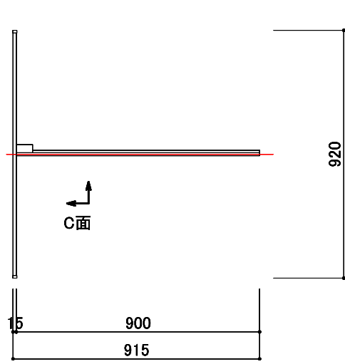
平面図 1/20
