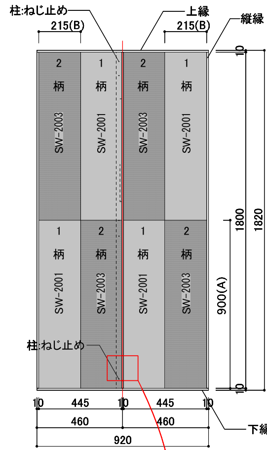
立面図 1/20
