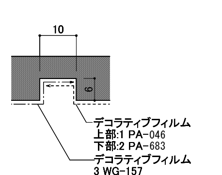
B部詳細図 1/1
