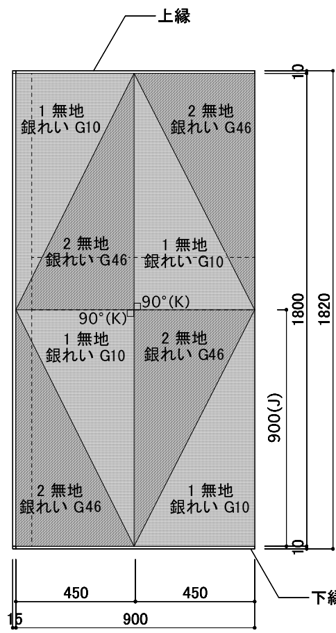
側面図 1/20
