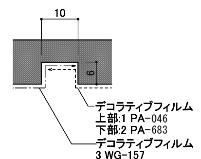
B部詳細図 1/1
