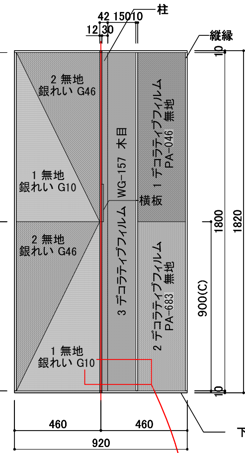
背面図 1/20
