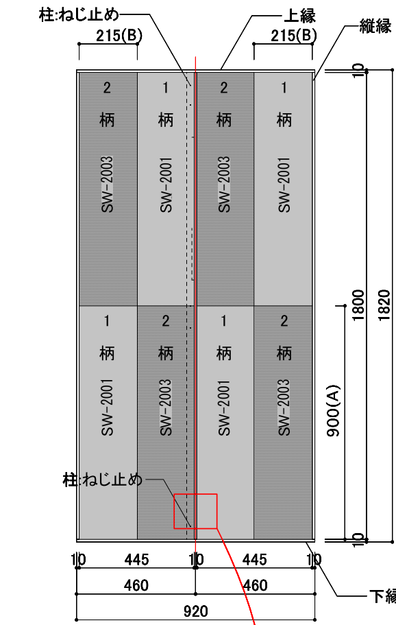
立面図 1/20
