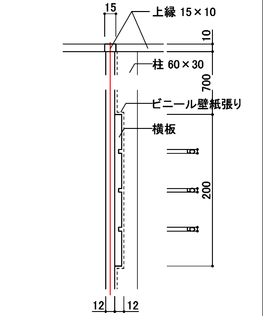
横板部断面図 1/5
