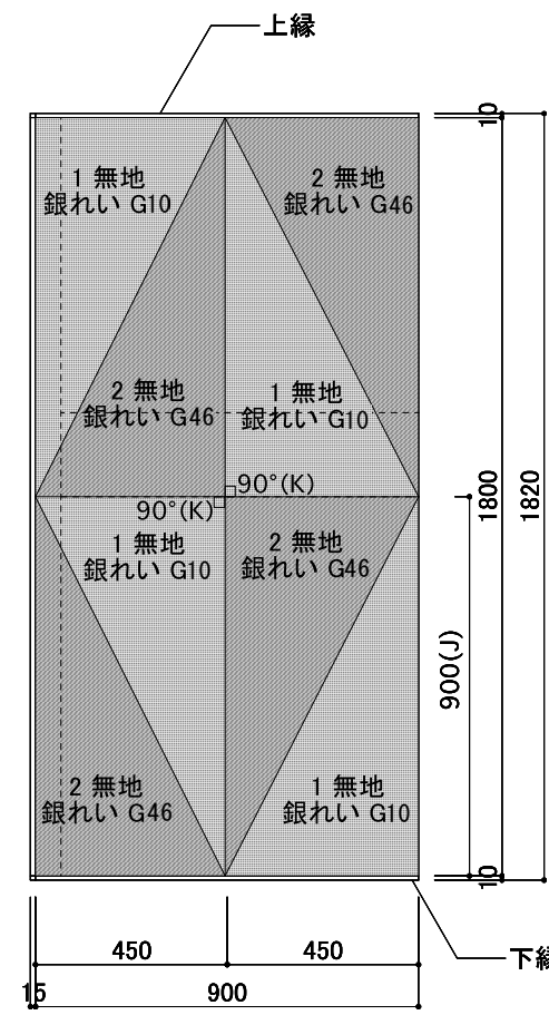
側面図 1/20
