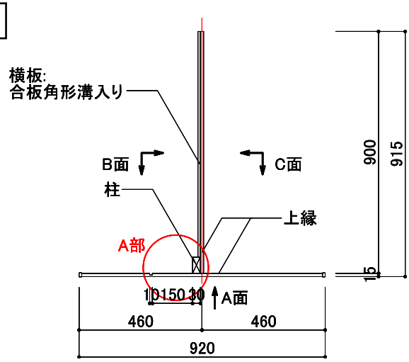
平面図 1/20
