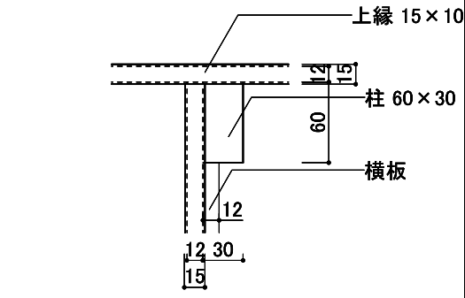
柱取合い部 伏図 1/5
