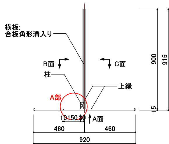
平面図 1/20
