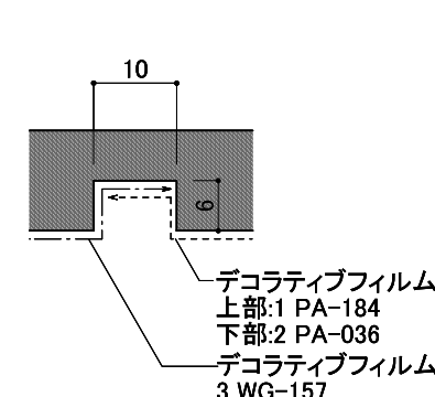
B部詳細図 1/1
