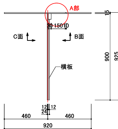
平面図 1/20
