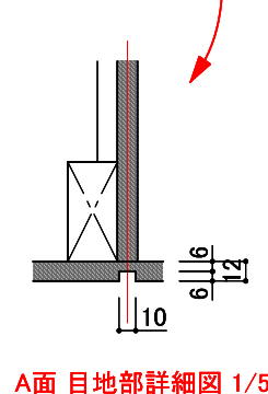
A面 目地部詳細図 1/5
