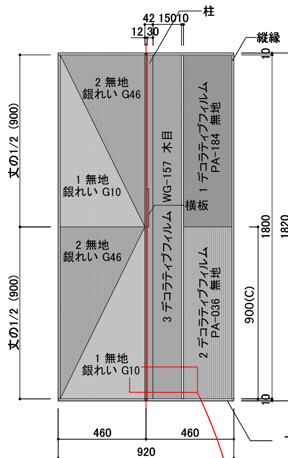
C面 紙壁紙 背面図 1/20
