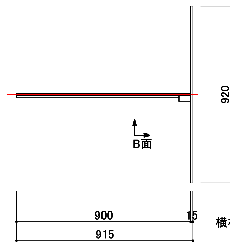
平面図 1/20
