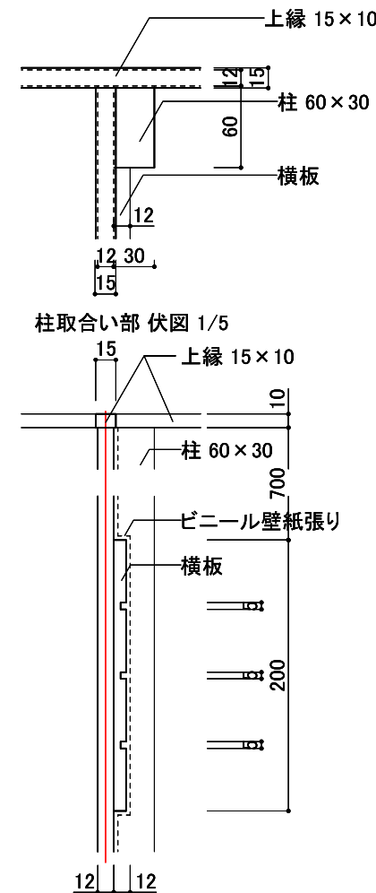
横板部断面図 1/5
