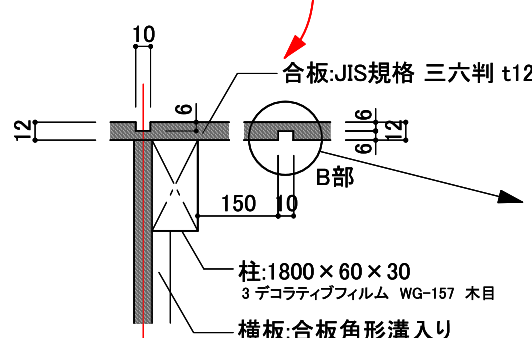
A部詳細図 1/5
