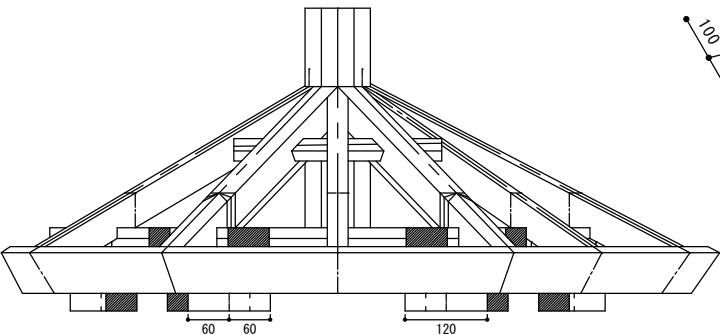
正面図
