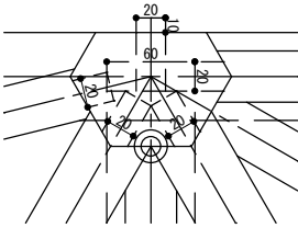
① 柱廻り詳細
