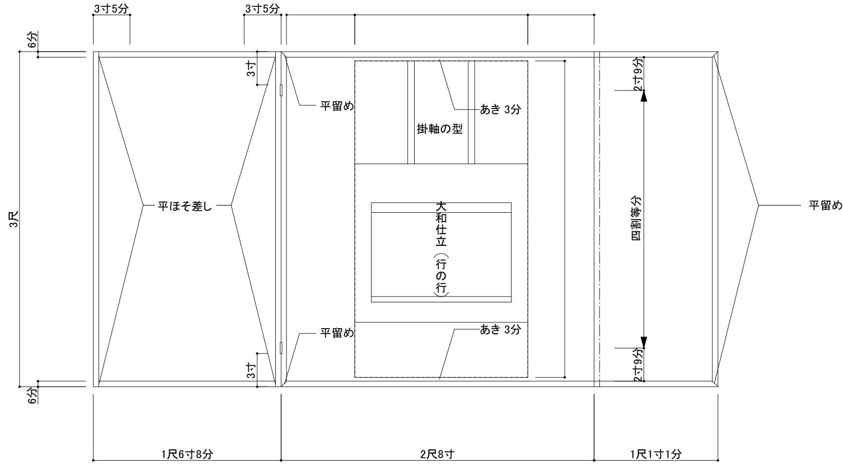
正面図 1/10
