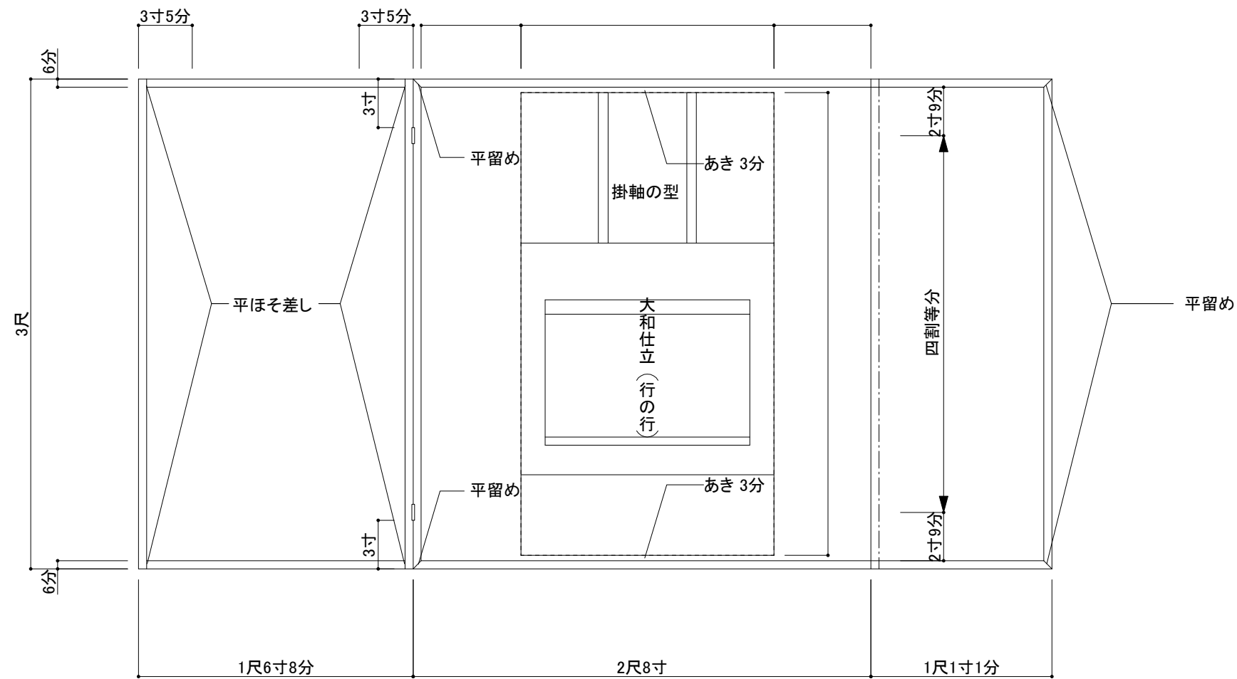
正面図 1/10
