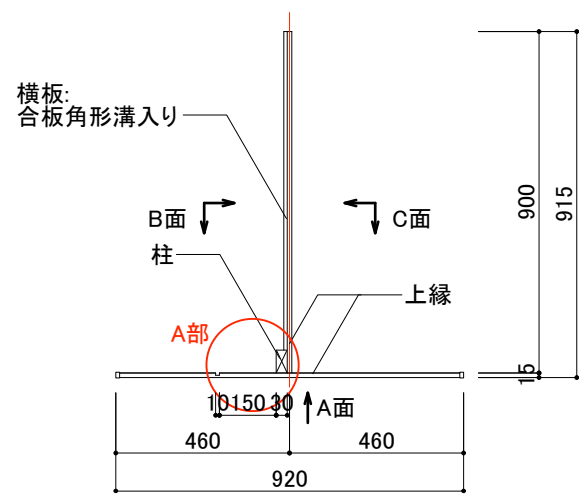
平面図 1/20
