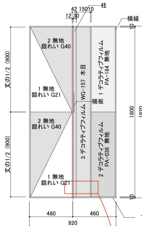
C面 紙壁紙 B面 デコラティブフィルム 背面図 1/20
