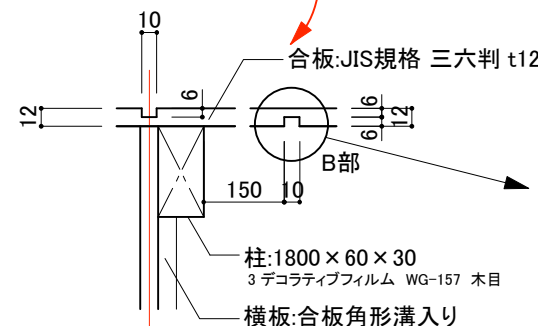
A部詳細図 1/5
