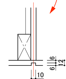
A面 目地部詳細図 1/5
