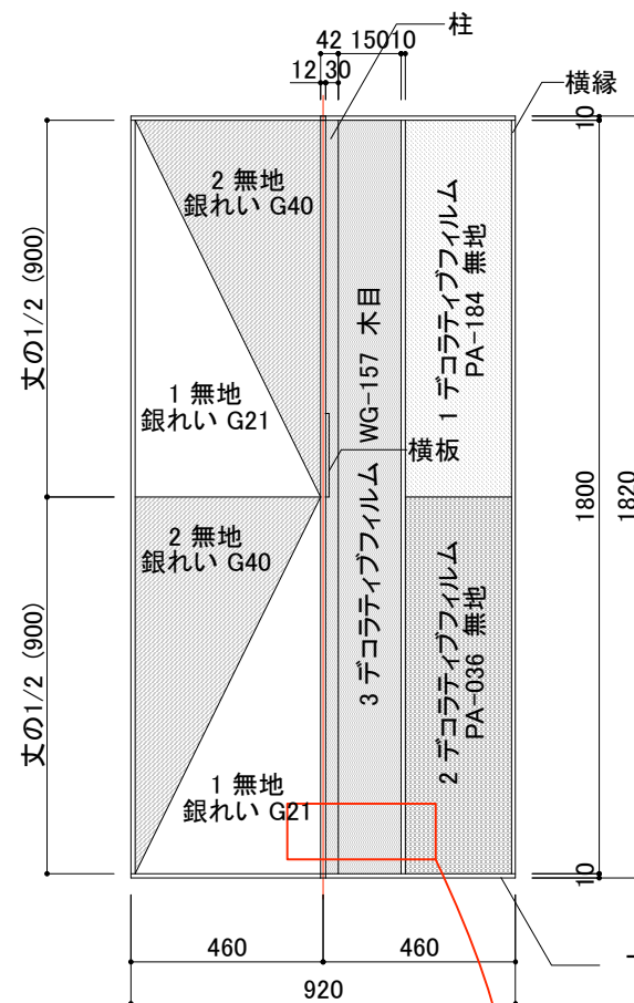
C面 紙壁紙 背面図 1/20
