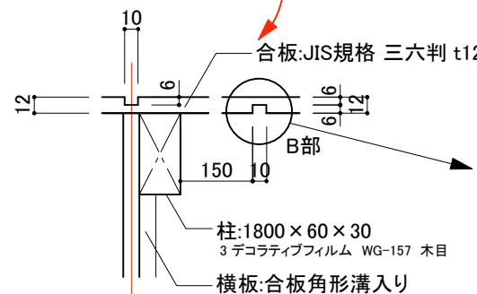
A部詳細図 1/5
