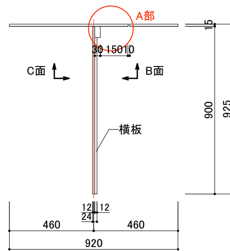
平面図 1/20
