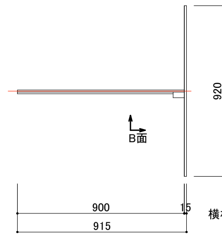
平面図 1/20
