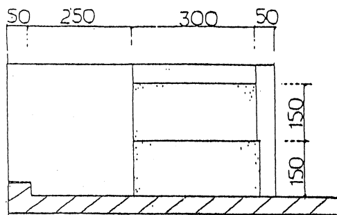
階段部(立面図)
