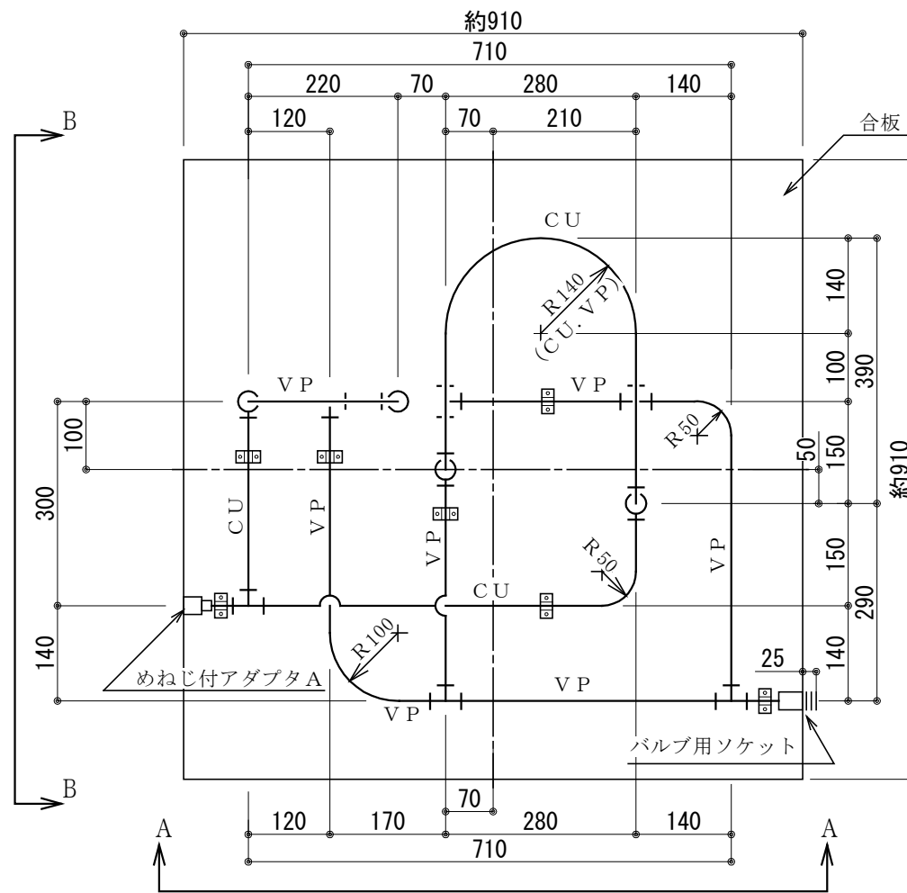
配管平面図 S : 1/10
