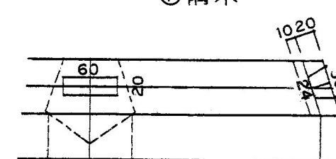
⑤ 梁
