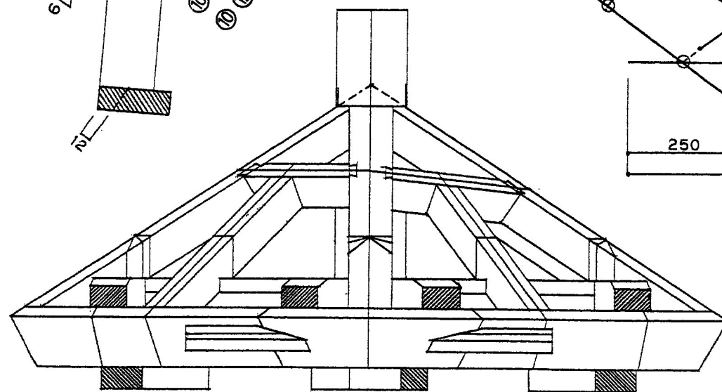
正面図
