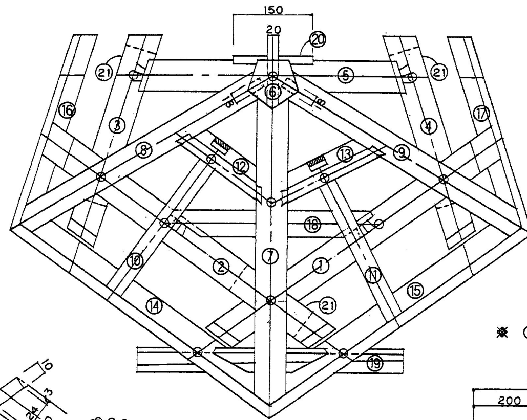
平面図
