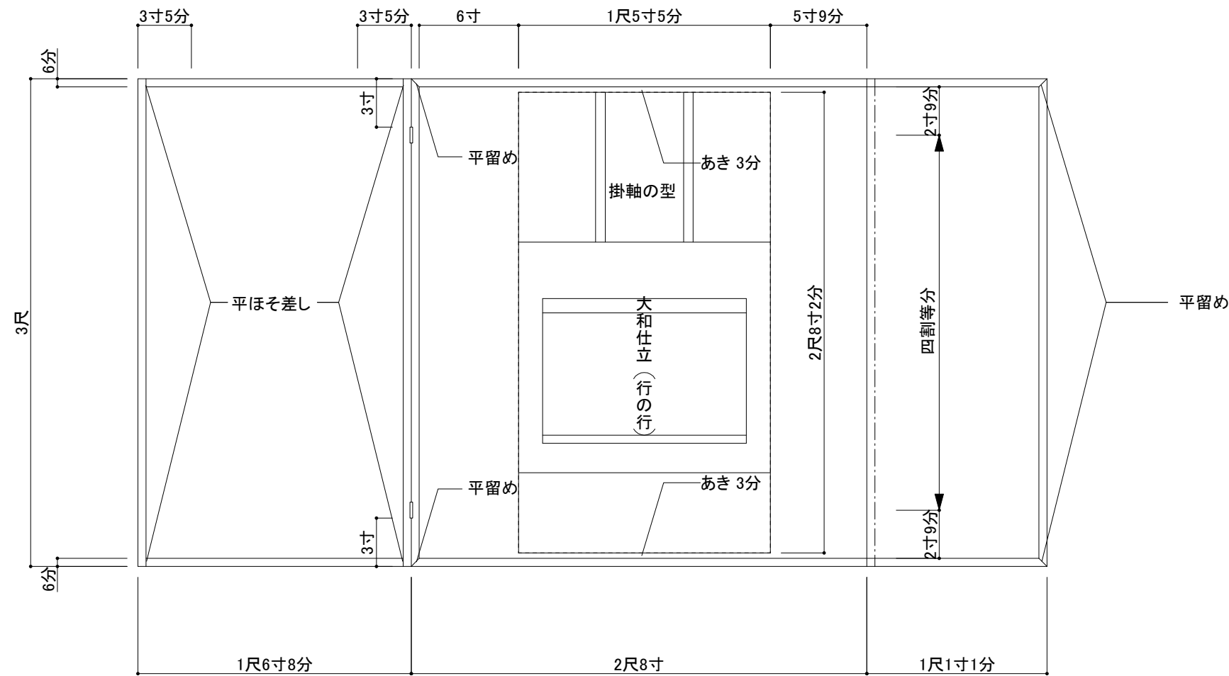
正面図 1/10
