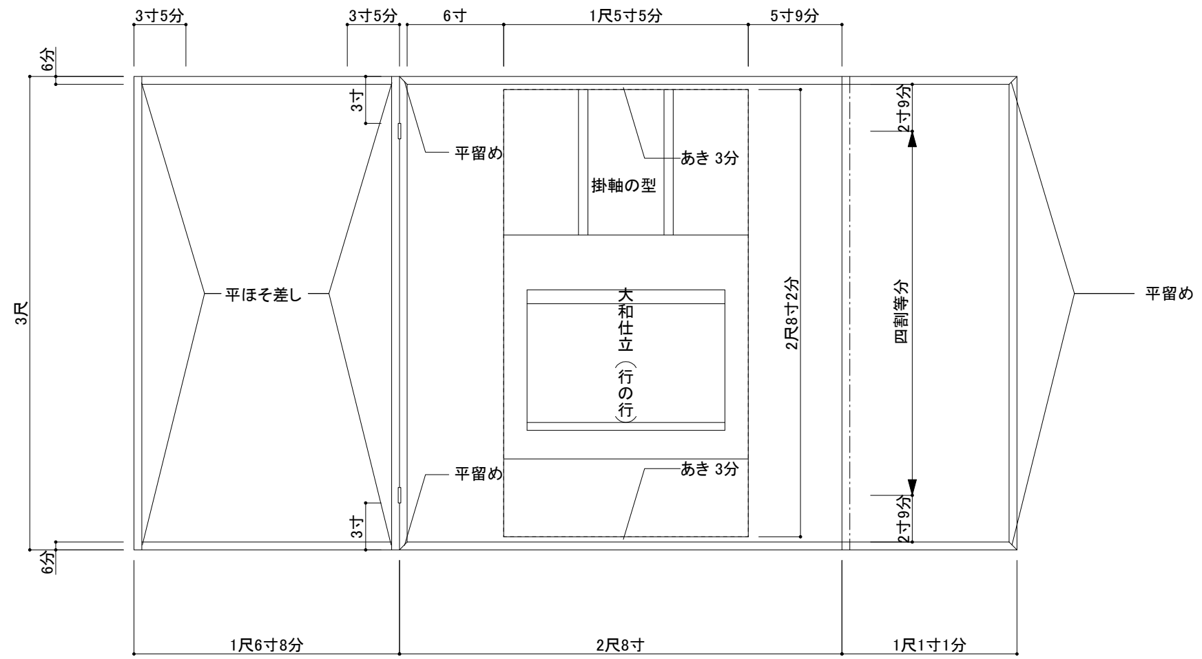
正面図 1/10
