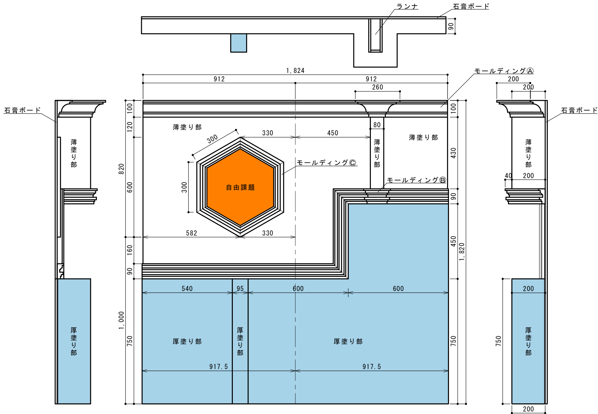
左官職種 1 - 1 競技課題図
