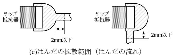
図 2 5 チップ抵抗器のはんだ付け基準
